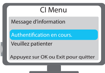
Phase d'authentification
